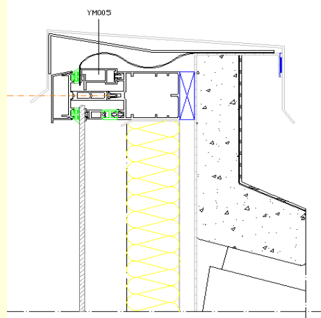
Raccord acrotère aspect grille
