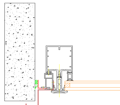
RACCORD MACONNERIE ASPECT TRAME HORIZONTALE:
