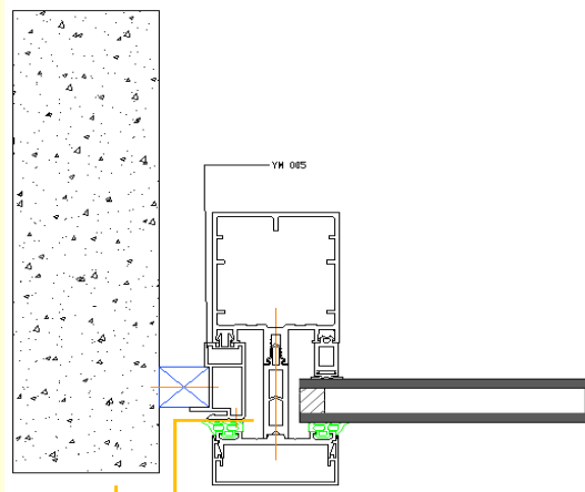
Raccord maçonnerie aspect grille
