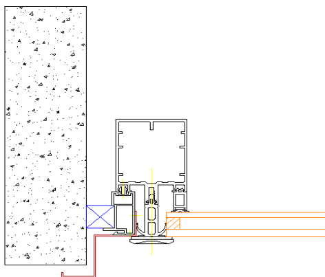
RACCORD MACONNERIE ASPECT TRAME HORIZONTALE:
