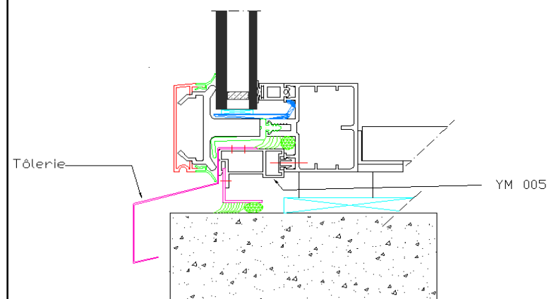
Raccord maçonnerie aspect grille (trame horizontale, serreur ponctuel)
