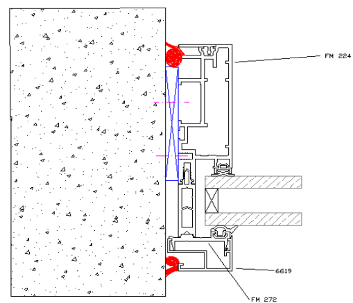
Liaison sur gros-oeuvre
