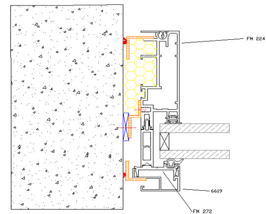
Liaison sur gros-oeuvre
