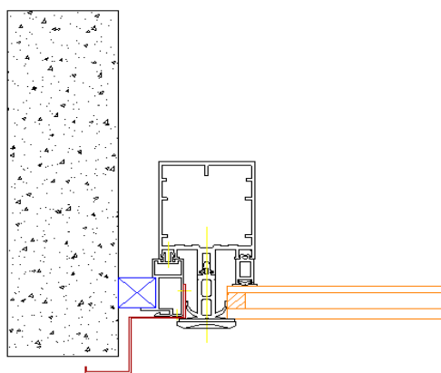
RACCORD MAÇONNERIE ASPECT TRAME HORIZONTALE:
