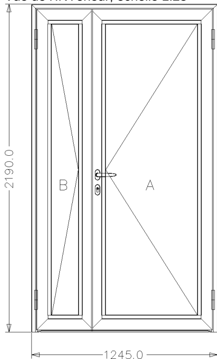
Vue de l'INTérieur, échelle 1:25
