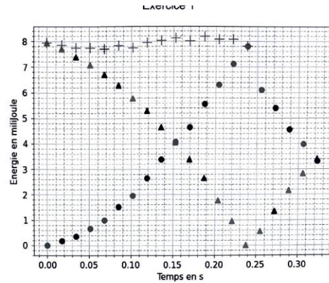
Figure 6 : évolutions des énergies mécanique, cinétique et potentielle de pesanteur de la balle lâchée depuis h = 30 cm
