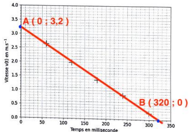
Figure 3 : évolution de la valeur de la vitesse de la balle en fonction du temps
