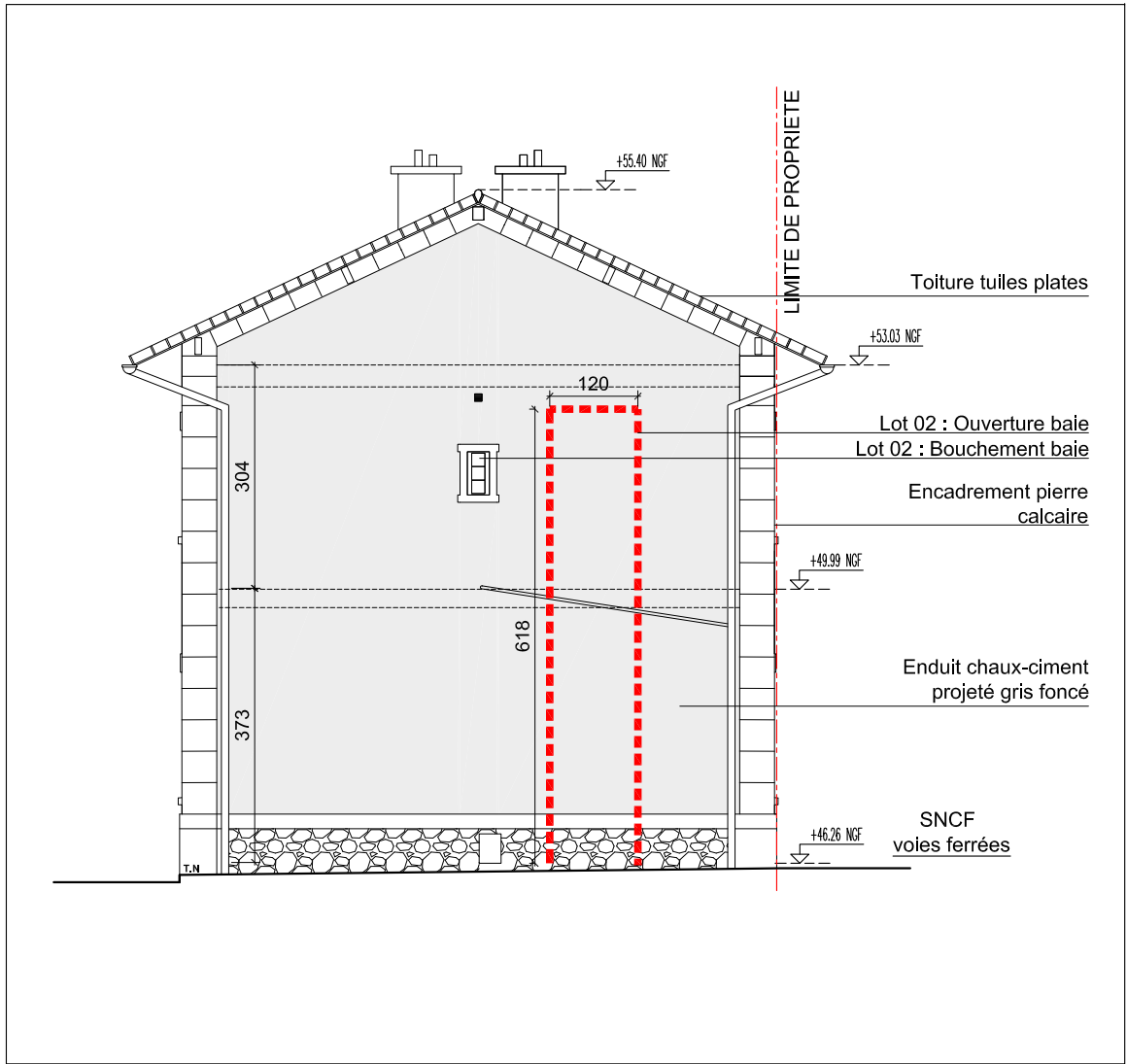
FACADE SUD EXISTANT Ech:1/100ème
