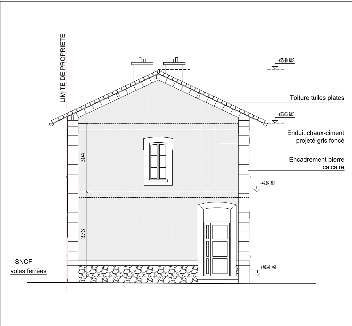
FACADE NORD EXISTANT Ech:1/100ème
