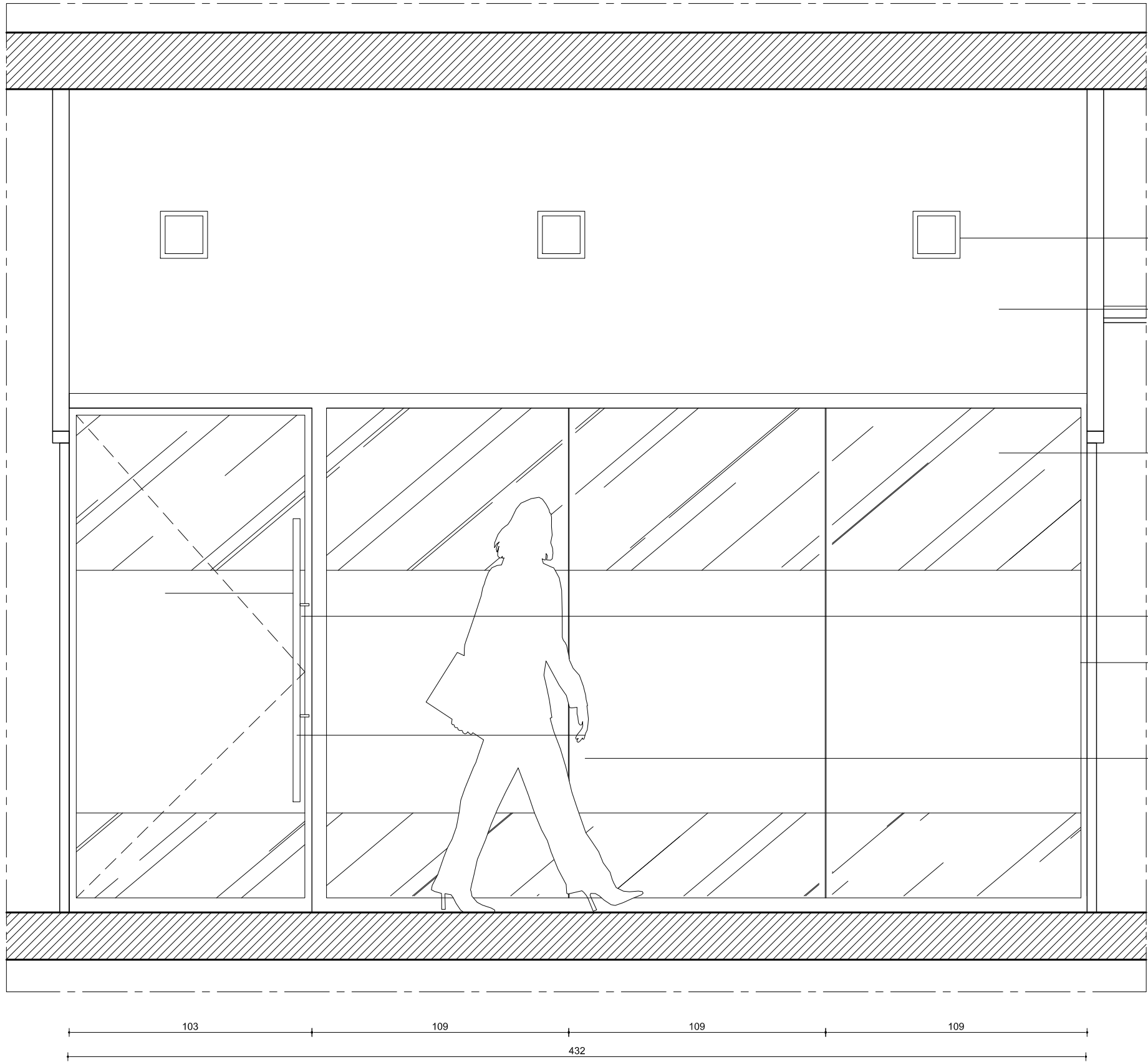
ELEVATION CLOISON VITREE Ech:1/20ème
