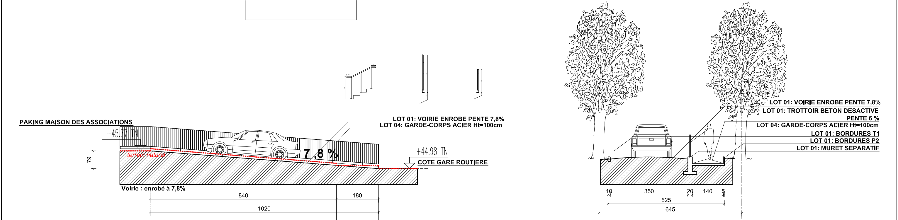
PROFIL EN TRAVERS VOIRIE et TROTTOIR Ech:1/100ème
