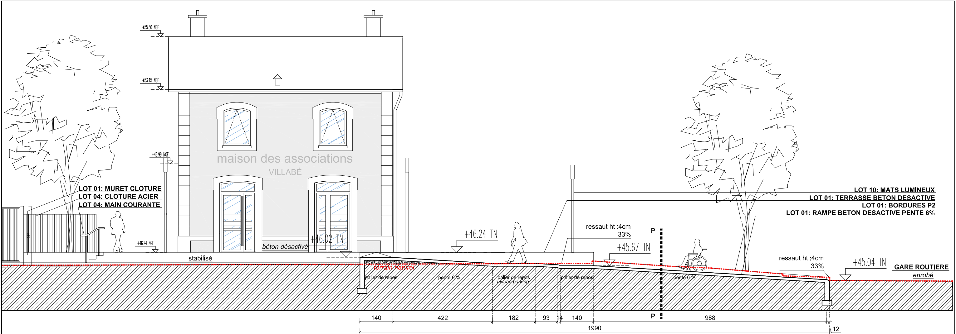
COUPE AA SUR TROTTOIR & RAMPE P.M.R Ech:1/100ème
