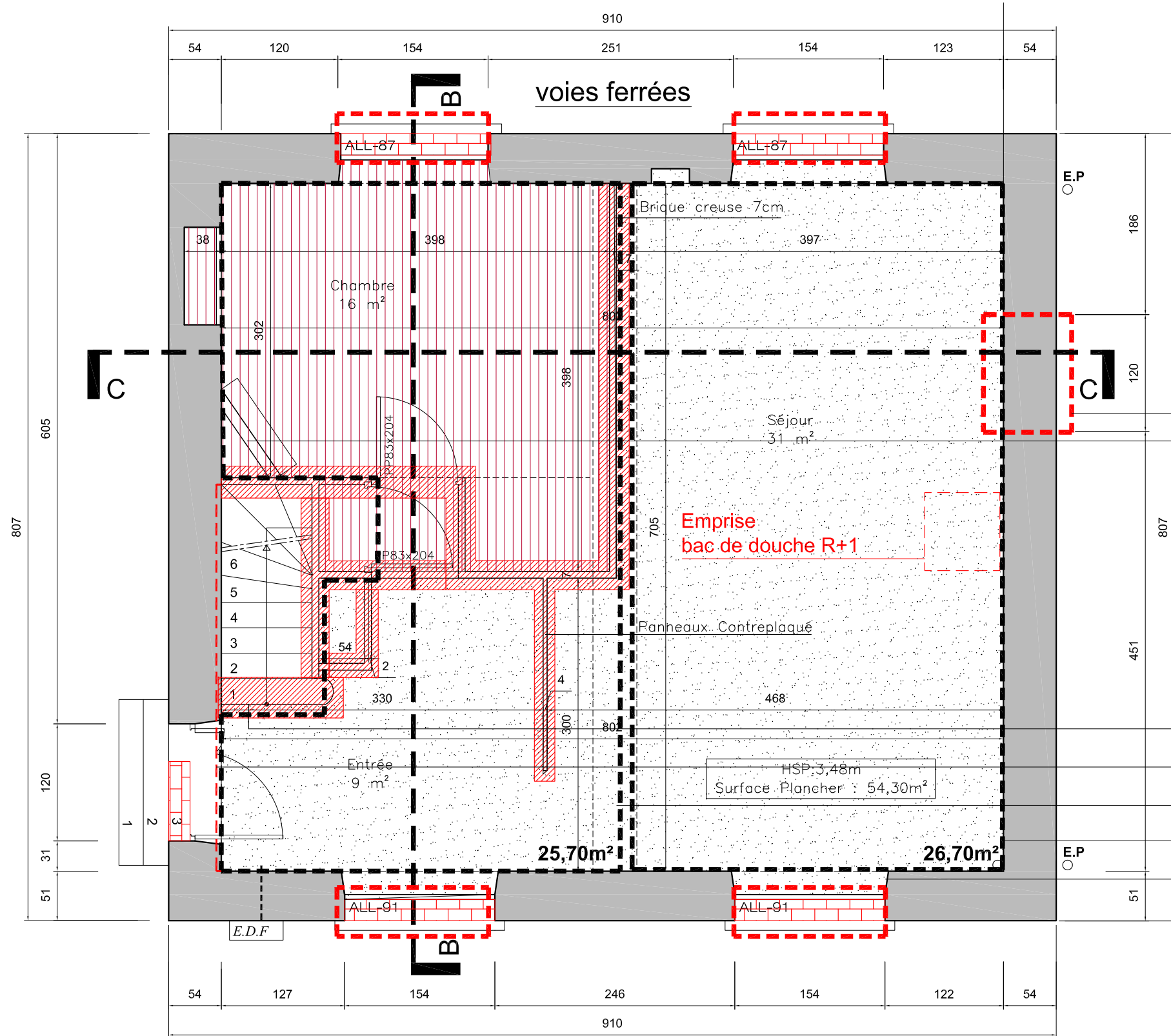
PLAN DU REZ-DE-CHAUSSEE EXISTANT
