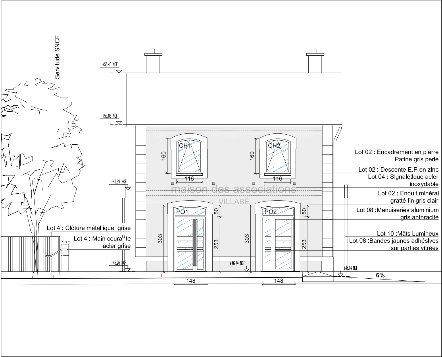
FACADE OUEST PROJET Ech:1/100ème
