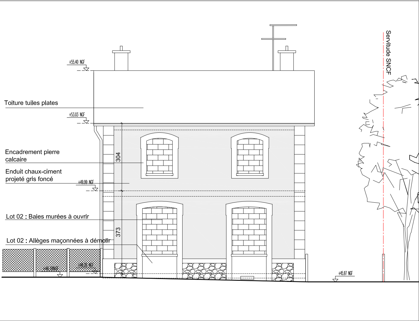
FACADE EST EXISTANT (côté voie ferrée ) Ech:1/100ème
