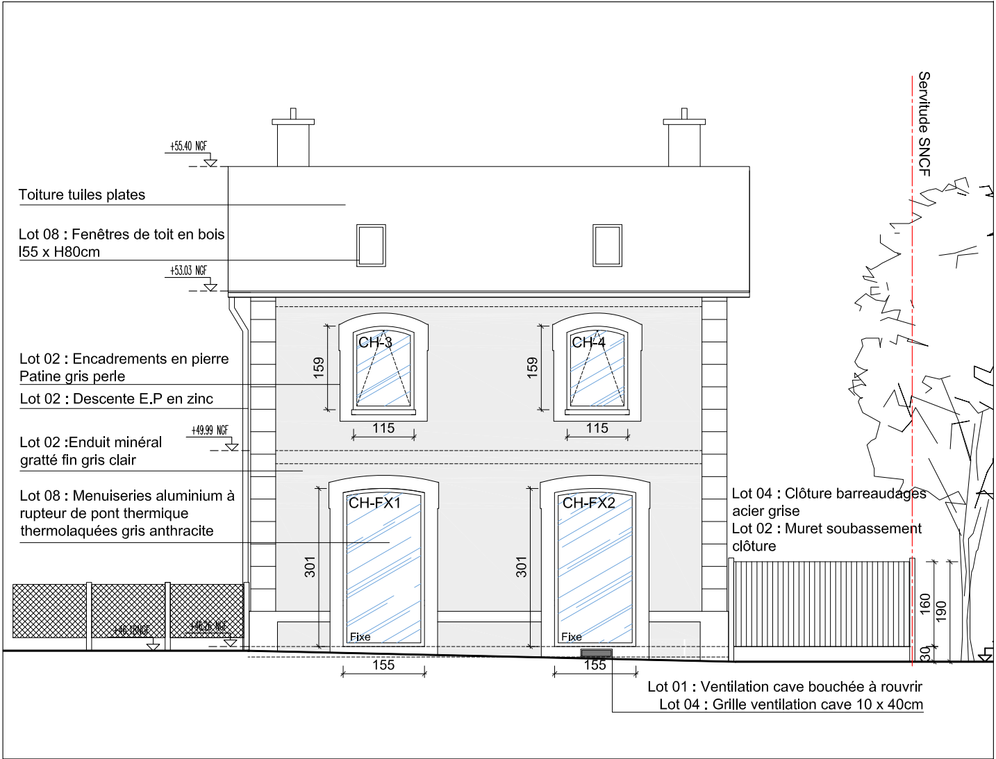
FACADE EST PROJET (côté voie ferrée) Ech:1/100ème
