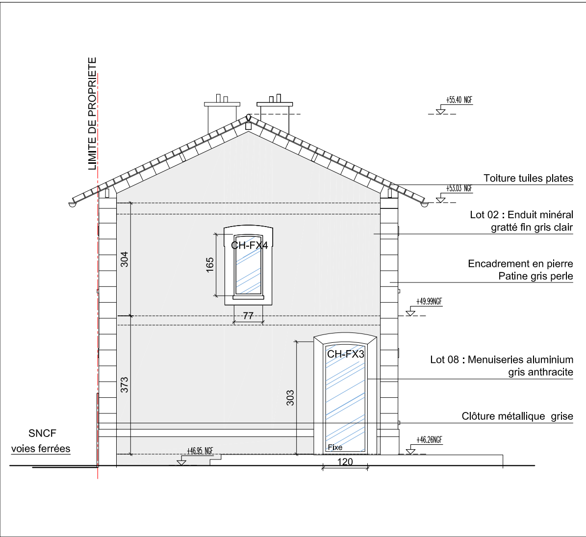
FACADE NORD PROJET Ech:1/100ème
