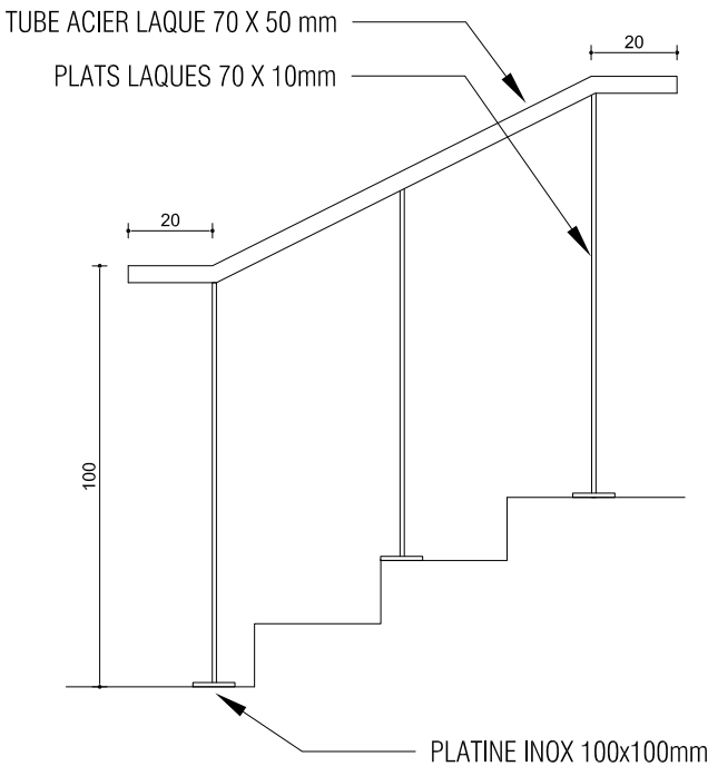
DETAIL MAINS COURANTES Ech:1/20ème
