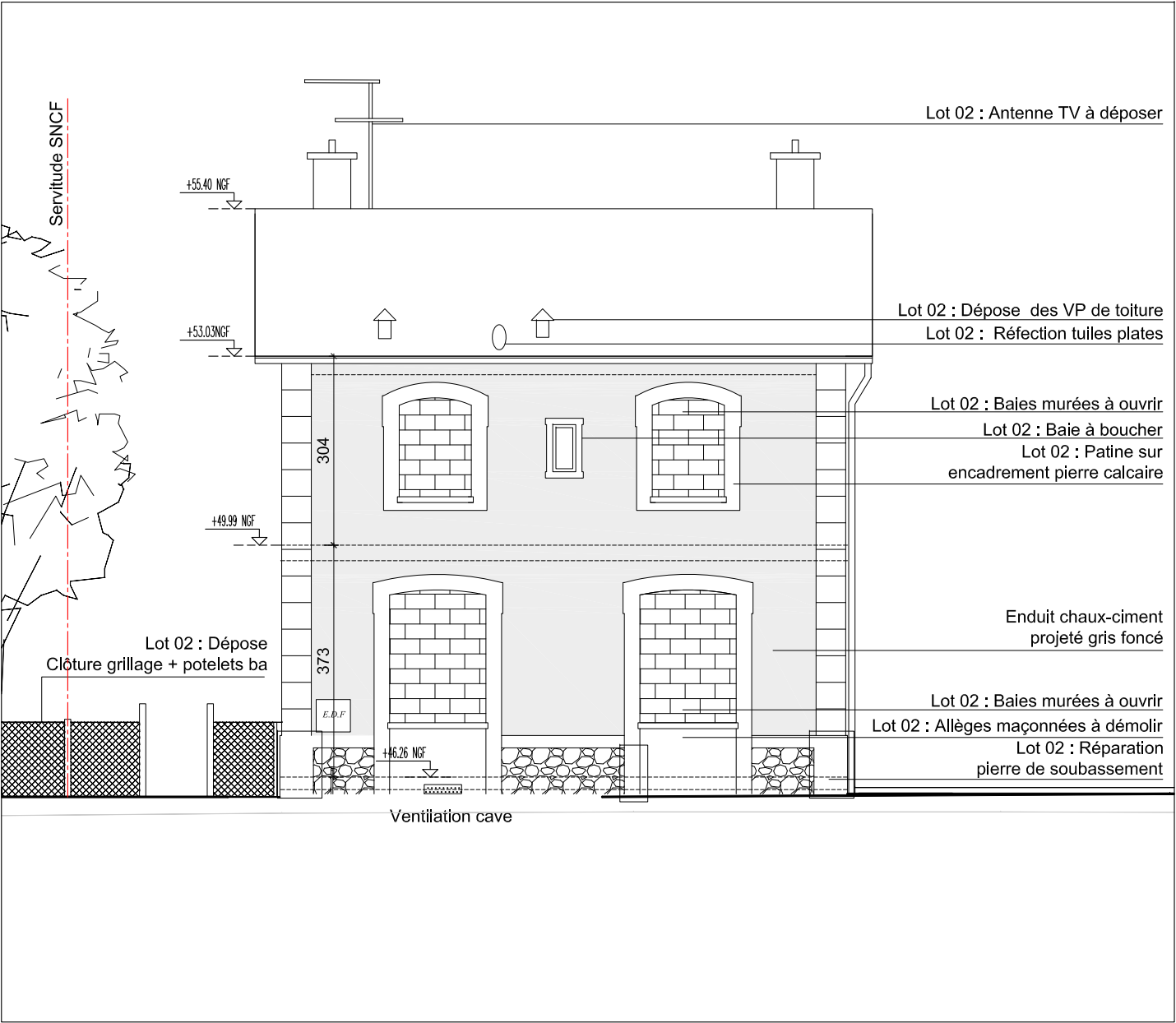
FACADE OUEST EXISTANT Ech:1/100ème
