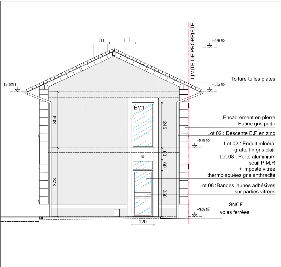
FACADE SUD PROJET Ech:1/100ème
