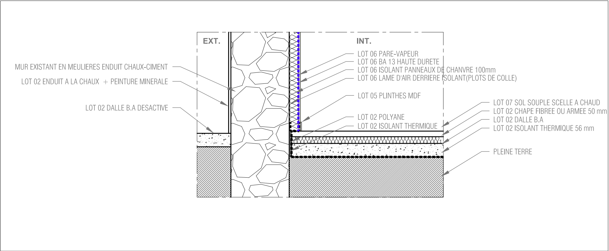
DETAIL ISOLATION Ech:1/10ème
