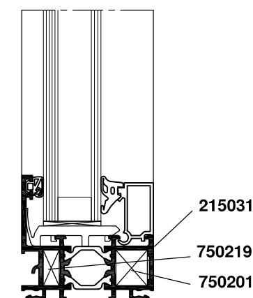
Variante dormant BTC drainage caché
