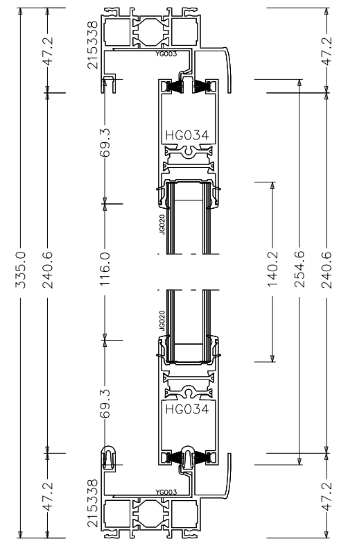
Coupe 2 B - B
