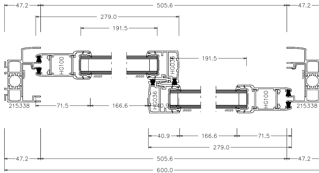
Coupe 1 A - A (Echelle : 1:2)
