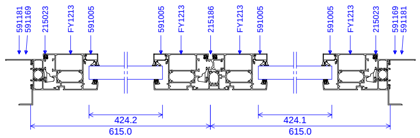
Coupe AA
