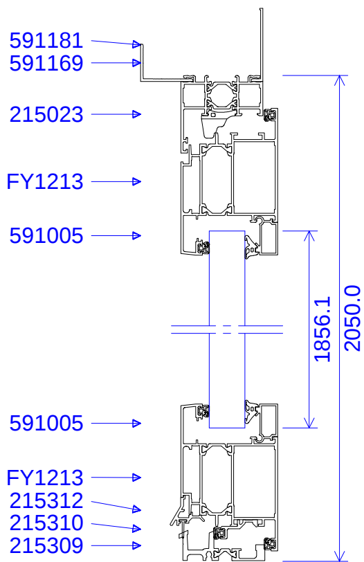
Coupe BB
