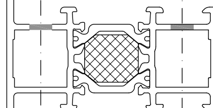
Assemblage avec 2 goupilles
